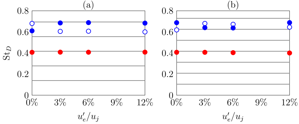
FIGURE 4.7 – Variations des nombres de Strouhal des pics ● dominants pour n_\theta = 0 et ○ dominants et ● secondaires pour n_\theta = 1 pour (a) L = 6r_0 et (b) L = 8r_0 avec le pic d'intensité des fluctuations de vitesse pour les jets libres équivalents; — nombres de Strouhal obtenus à partir du modèle (4.1).
