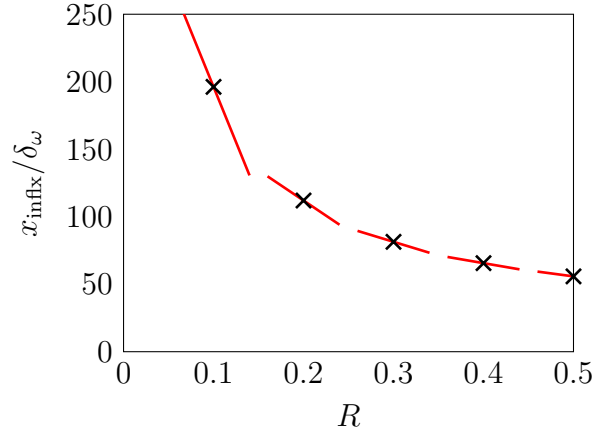
FIGURE 3.6 – Variations \times des positions des points d'inflexion dans les profils des valeurs quadratiques moyennes des fluctuations de vitesse transverse et — de leurs dérivées vis-à-vis du rapport de vitesse.
