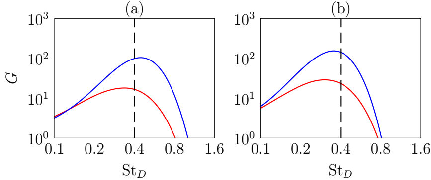
FIGURE 4.10 – Gains en amplitude des ondes d’instabilité entre z = 0 et z = L - r_0 pour n_\theta = 0 pour les jets (a) — 0%L6 et — 12%L6, et (b) — 0%L8 et — 12%L8 ; — — — nombre de Strouhal du pic dominant dans les spectres acoustiques.
