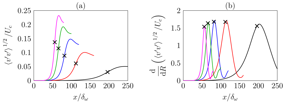
FIGURE 3.4 – Variations en y = 0 (a) des valeurs quadratiques moyennes des fluctuations de vitesse transverse et (b) de leurs dérivées vis-à-vis du rapport de vitesse pour — R = 0.1 , — R = 0.2 , — R = 0.3 , — R = 0.4 et — R = 0.5 ; \times points d'inflexion dans les profils des valeurs quadratiques moyennes des fluctuations de vitesse.
