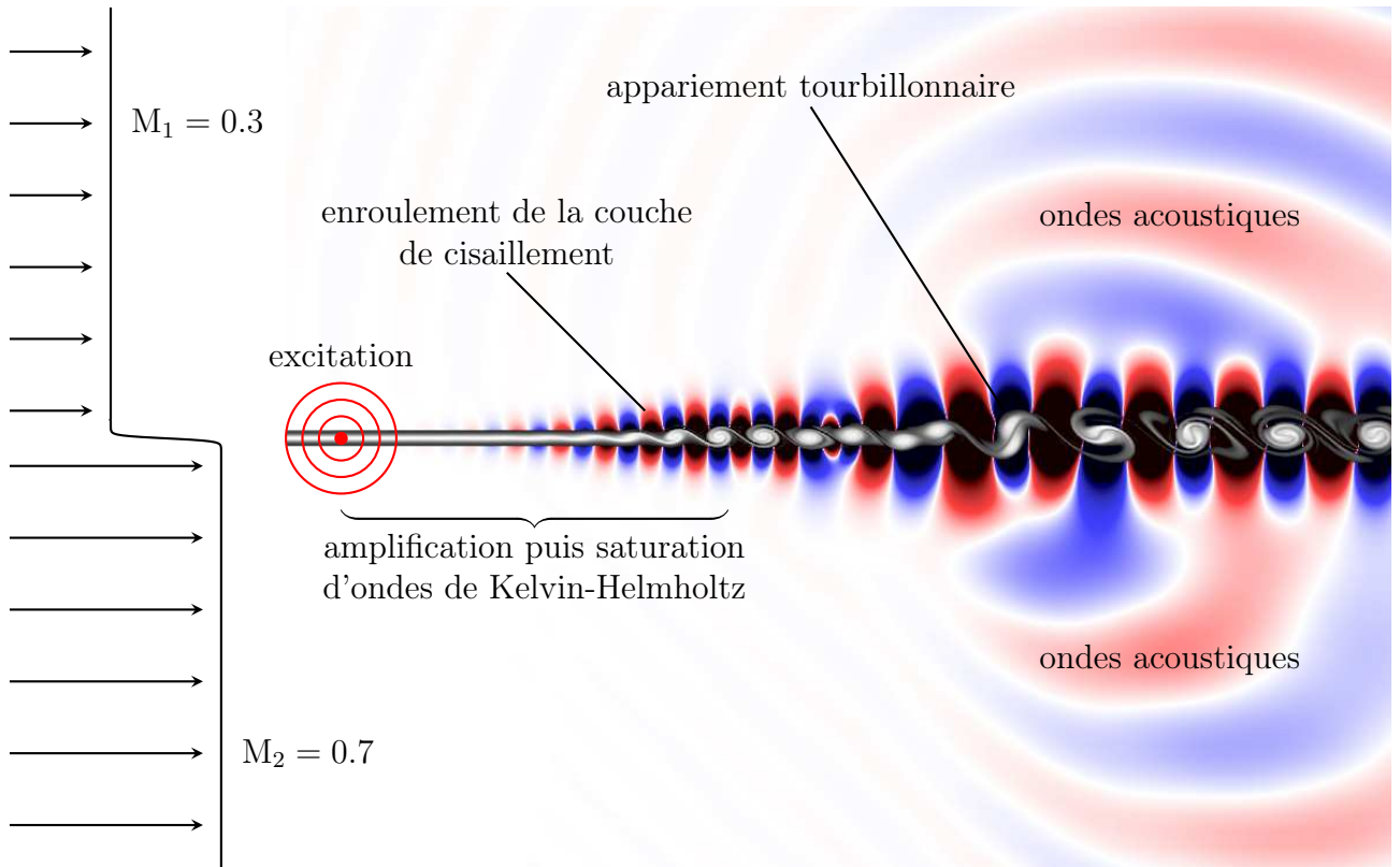
FIGURE 1.4 – Représentation du développement aérodynamique et du rayonnement acoustique d'une couche de mélange bidimensionnelle contrôlée par une excitation harmonique.
