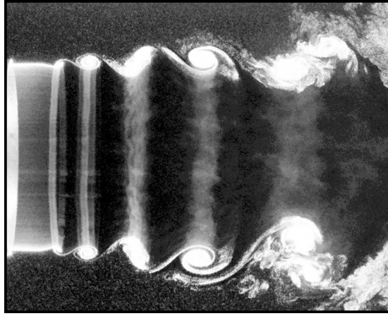
FIGURE 1.2 – Visualisation par fumée d'un jet rond d'air avec des couches limites laminaires excitées à une fréquence ; d'après Schram [255] ; vitesse d'éjection u_j \simeq 34 \text{ m.s}^{-1} , nombre de Reynolds Re_D = 93000 et nombres de Strouhal associés à l'excitation St_\theta = 0.013 et St_D = 3 .
