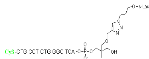
Glycoconjugate 23 (G 23)
