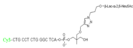
Glycoconjugate 24 (G 24)
