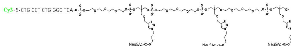
Glycoconjugate 19 (G 19)
