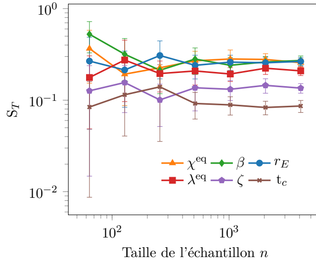
FIG. E.2 : Étude de convergence de la taille de l'échantillon n sur l'indice du première ordre S_T à t = 20 jours pour les six paramètres les plus influents sur la sortie S_i^\dagger .
