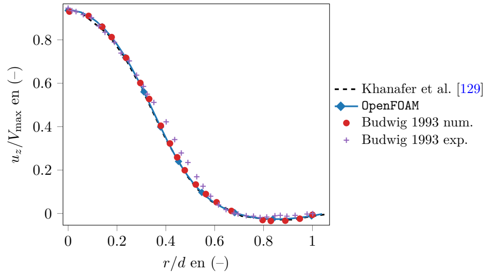
FIG. G.3 : Validation en géométrie anévrismale par comparaison avec Khanafer et al. [129, Fig. 4] écoulement à Re = 400 . Les données initiales de Ahmed et Giddens [3] sont également reportées après numérisation.
