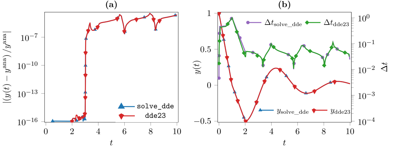
FIG. B.1 : Validation de solve_dde sur l'EDR (B.1.1) et comparaison avec dde23 . (a) : Erreur relative de l'intégration numérique par rapport à la solution analytique. (b) : Ordonnée de gauche : évolution temporelle de y . Ordonnée de droite : variation des pas de temps choisis par les algorithmes en échelle logarithmique.
