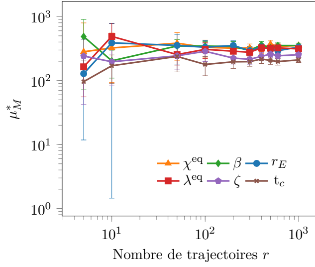
FIG. E.1 : Étude de convergence du nombre de trajectoires considérées r sur \mu_M^* à t = 20 jours pour les six paramètres les plus influents sur la sortie S_i^\dagger .
