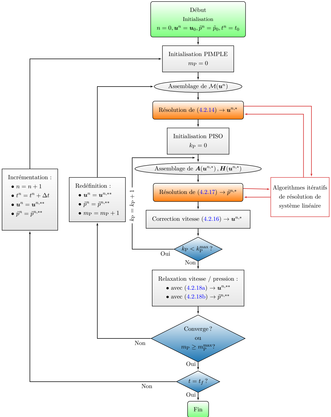
FIG. 4.6 : Organigramme de l'algorithme PIMPLE implémenté dans OpenFOAM . On représente : les résolutions des systèmes linéaires par des encarts rectangulaires orange, les assemblages de matrices par des ellipses grises, les conditions par des losanges bleus, et les évaluations par des encarts rectangulaires gris. Initialement, l'algorithme demande les conditions initiales du problème. Pour chaque pas de temps, une solution stationnaire est recherchée grâce à une boucle PIMPLE qui combine les étapes d'un SIMPLE dans laquelle une boucle PISO est réalisée un nombre k_P^{\max} de fois. Après convergence de la boucle PIMPLE ou dépassement du nombre maximale de cycles PIMPLE m_P^{\max} , l'algorithme avance en temps et réitère une boucle PIMPLE jusqu'à atteindre le temps final t_f .
